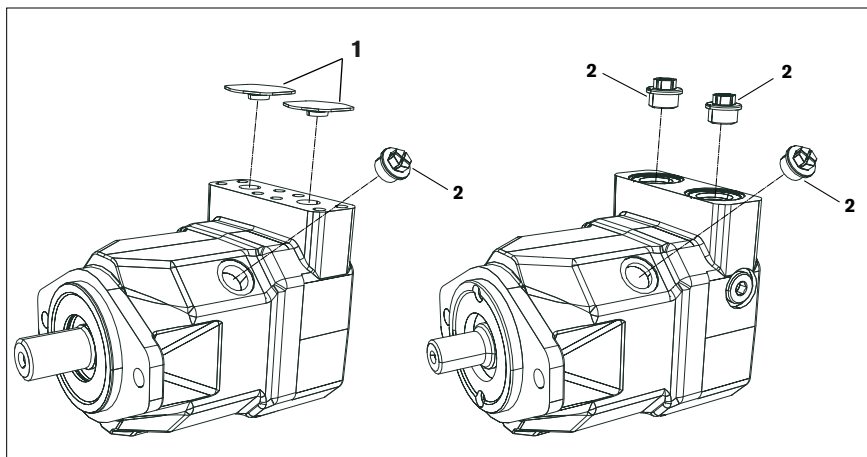
Abb. 9: Transportschutz entfernen
