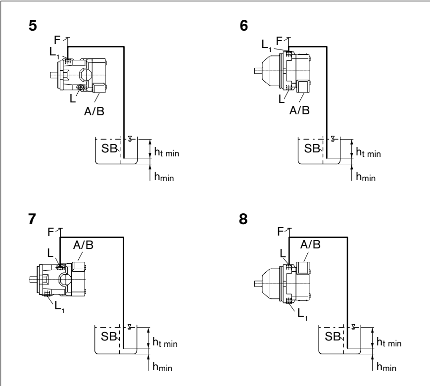
Abb. 7: Übertankeinbau A10FM mit Einbaulage 5–8
