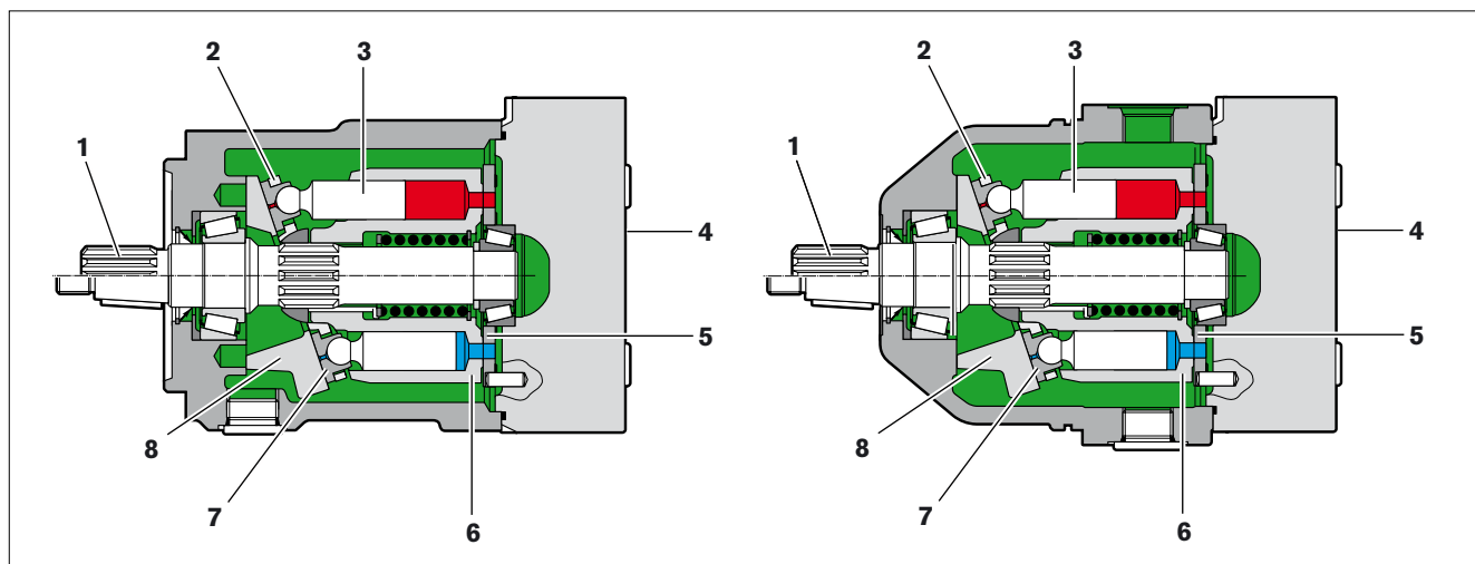
Abb. 2: Aufbau der A10FM (linke Darstellung) und A10FE (rechte Darstellung)
