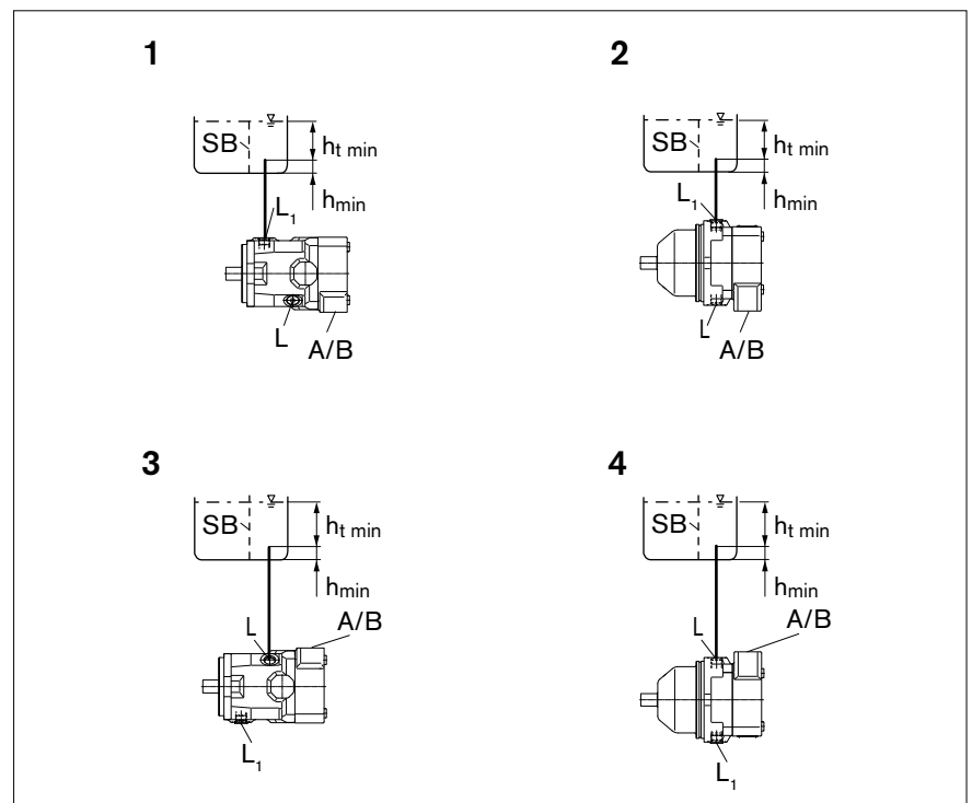
Abb. 6: Untertankeinbau A10FM/A10FE mit Einbaulage 1–4
