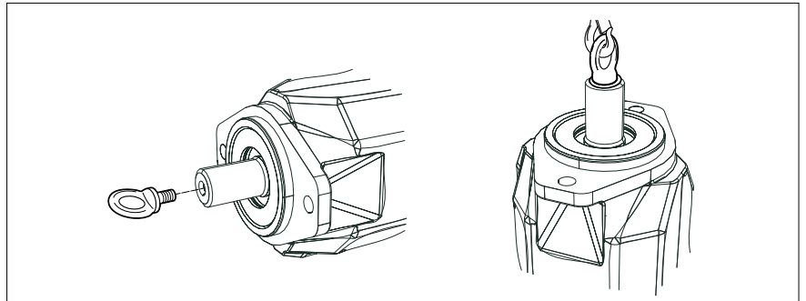
Abb. 4: Befestigung der Ringschraube
