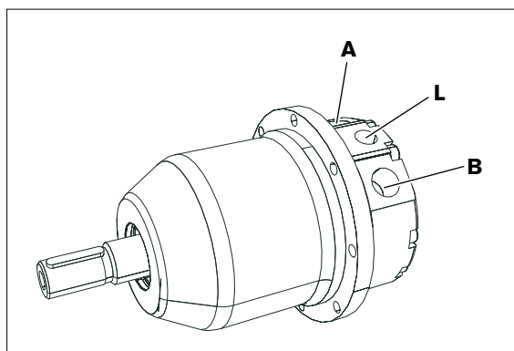
Abb. 14: Anschlussübersicht A10FE mit speziell 8-Loch-Anbauflansch H, Nenngröße 11 bis 18
