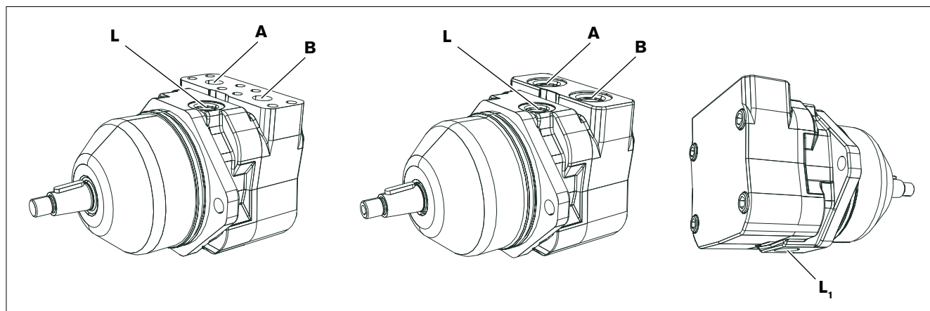
Abb. 11: Anschlussübersicht A10FE, linke Darstellung mit SAE-Flanschanschluss (Anschlussplatte 10), rechte Darstellung mit Gewindeanschluss (Anschlussplatte 16), Nenngröße 23 bis 45
