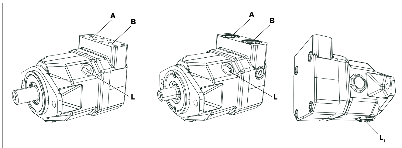
Abb. 10: Anschlussübersicht A10FM, linke Darstellung mit SAE-Flanschanschluss (Anschlussplatte 10), mittlere Darstellung mit Gewindeanschluss (Anschlussplatte 16)
