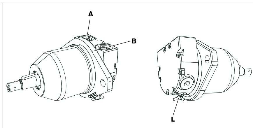
Abb. 13: Anschlussübersicht A10FE mit SAE 2-Loch-Anbauflansch C, Nenngröße 10 bis 18
