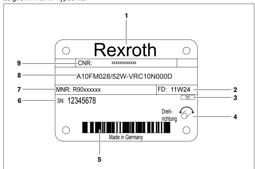
Abb. 3: Typschild A10FM
