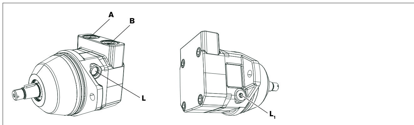
Abb. 12: Anschlussübersicht A10FE, Nenngröße 58 bis 63
