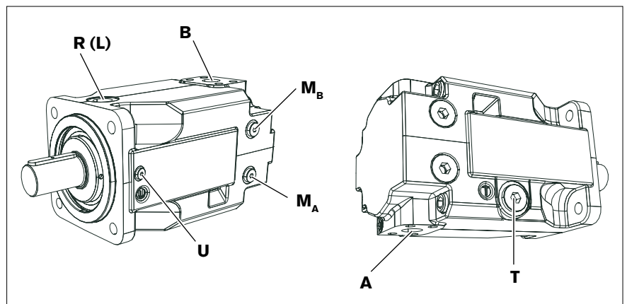
Abb. 14: Anschlussübersicht A4FM, Nenngröße 125 bis 500, SAE Flanschanschlüsse seitlich gegenüberliegend (Anschlussplatte 02)
