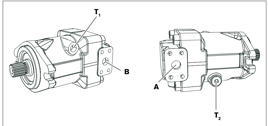
Abb. 12: Anschlussübersicht A4FM, Nenngröße 22 bis 40, SAE Flanschanschlüsse seitlich gegenüberliegend (Anschlussplatte 02)
