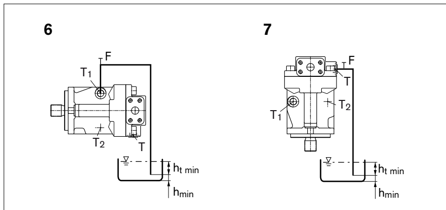
Abb. 8: Übertankeinbau für Nenngroße 22 bis 56 mit Einbaulage 6–7
