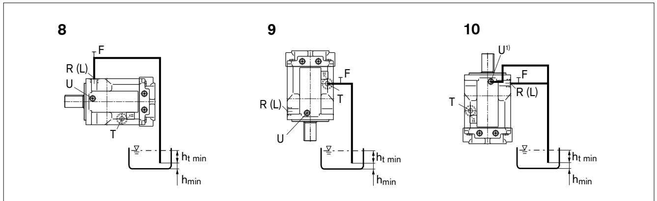
Abb. 9: Übertankeinbau für Nenngröße 71 bis 500 mit Einbaulage 8–10
