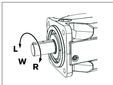
Abb. 10: Drehrichtung
