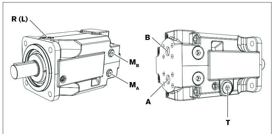
Abb. 13: Anschlussübersicht A4FM, Nenngröße 71, SAE Flanschanschlüsse hinten (Anschlussplatte 01)
