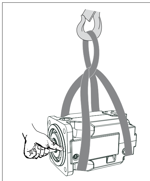
Abb. 5: Transport mit Hebeband
