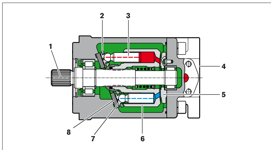
Abb. 2: Aufbau der und A4FM
