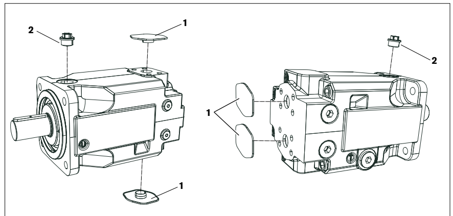
Abb. 11: Transportschutz entfernen
