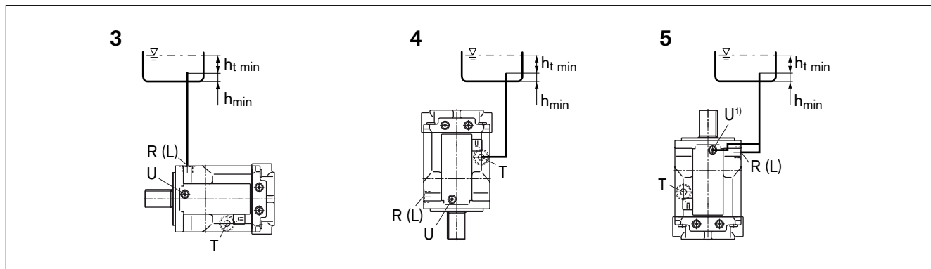
Abb. 7: Untertankeinbau für Nenngroße 71 bis 500 mit Einbaulage 3–5
