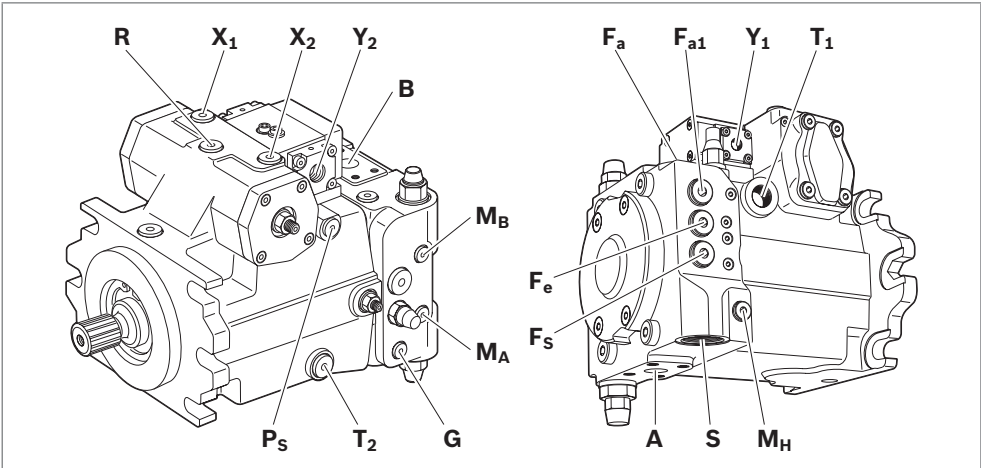
Abb. 16: Anschlussübersicht A4VG, Nenngröße 71 bis 180
