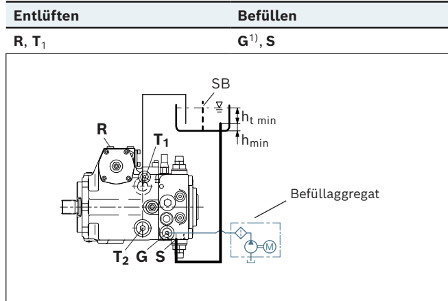
Einbaulage 1
