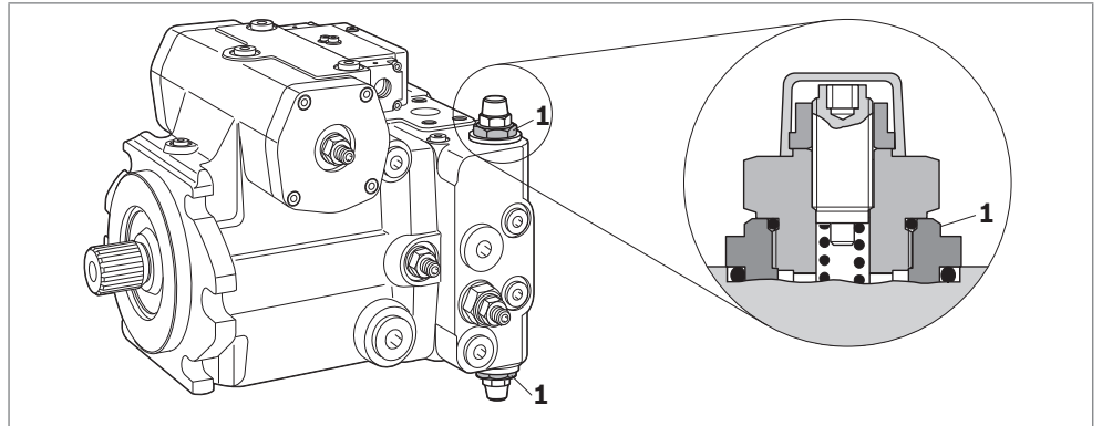
Abb. 5: Bypass-Funktion Nenngroße 125 bis 180 aktivieren
