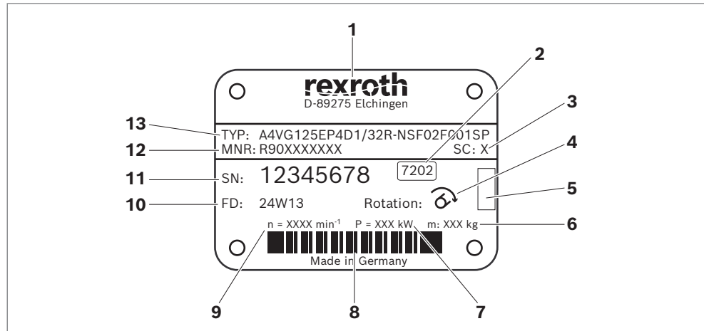
Abb. 6: Typschild A4VG
