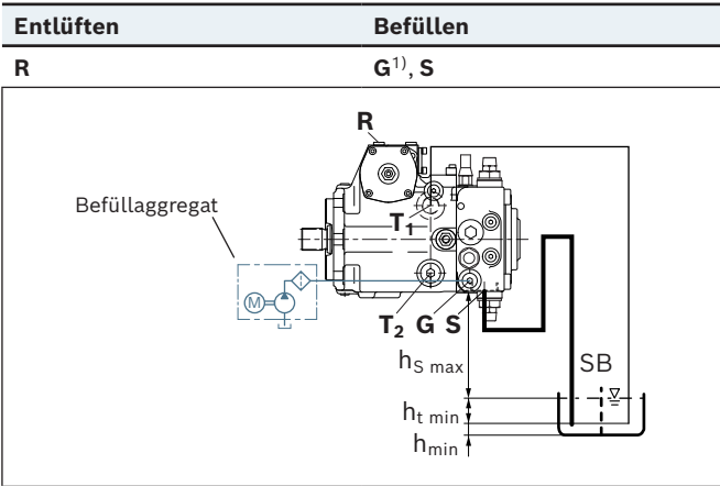
Einbaulage 7
