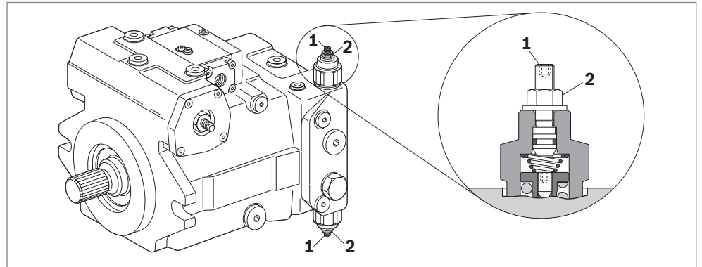
Abb. 3: Bypass-Funktion Nenngroße 28 bis 56 aktivieren
