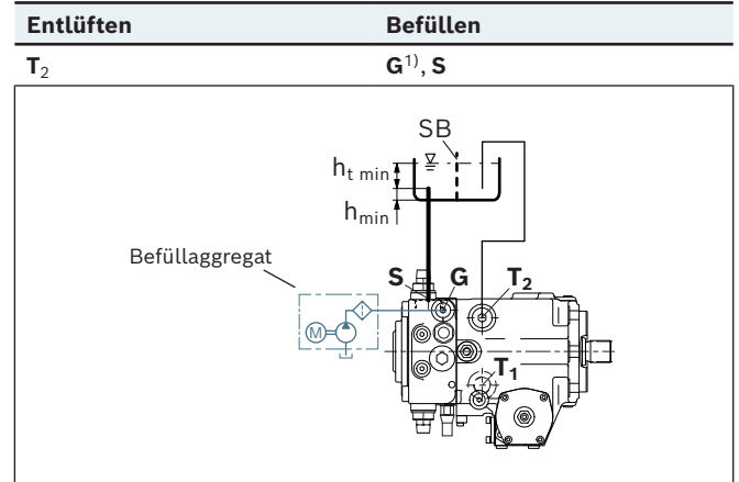
Einbaulage 2
