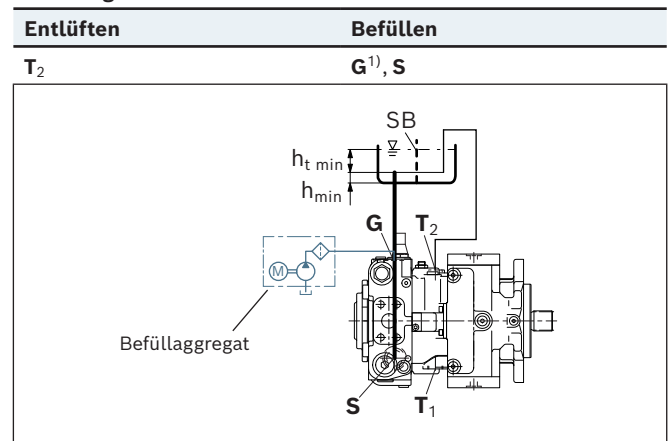
Einbaulage 6
