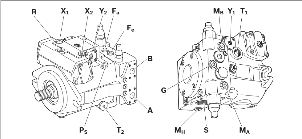
Abb. 14: Anschlussübersicht A4VG, Nenngröße 28
