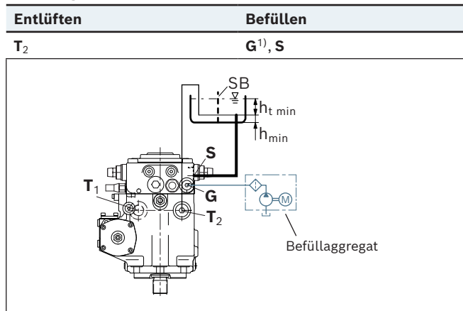
Einbaulage 3
