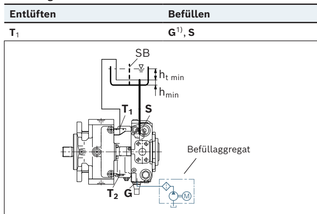
Einbaulage 5
