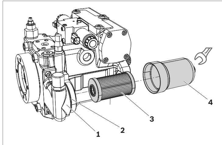
Abb. 18: Filterelement wechseln von Anbaufilter
