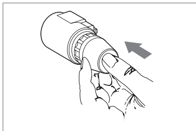
Abb. 17: Manuelle Übersteuerung bei elektrischer Proportionalverstellung
