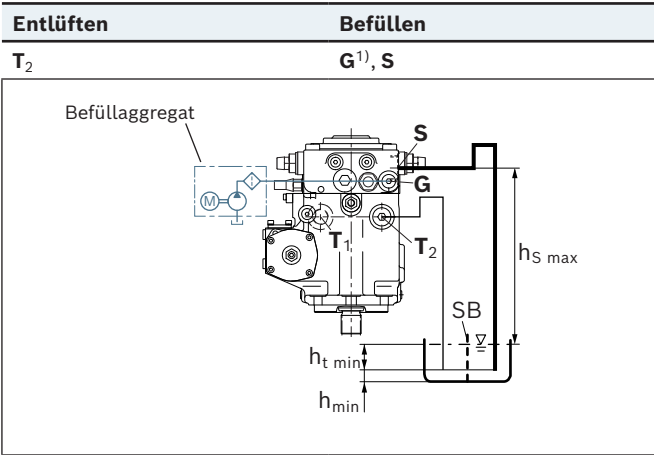
Einbaulage 9
