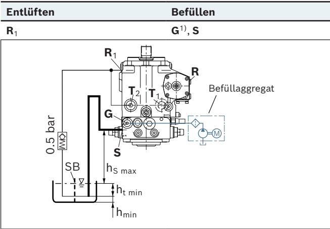
Einbaulage 10
