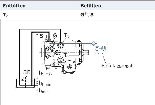
Einbaulage 8
