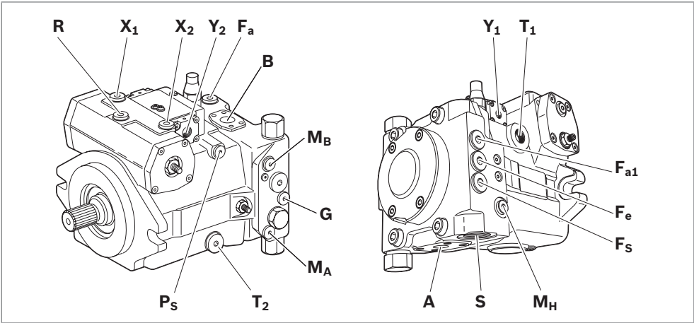
Abb. 15: Anschlussübersicht A4VG, Nenngröße 40, 56
