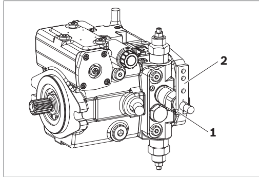
Abb. 13: Hebelposition von DA-Regelventil ändern
