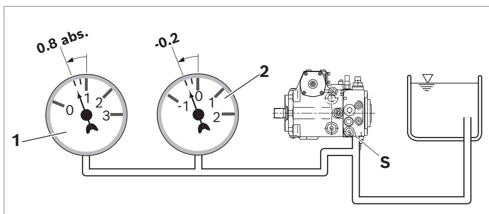
Abb. 9: Saugdruck
