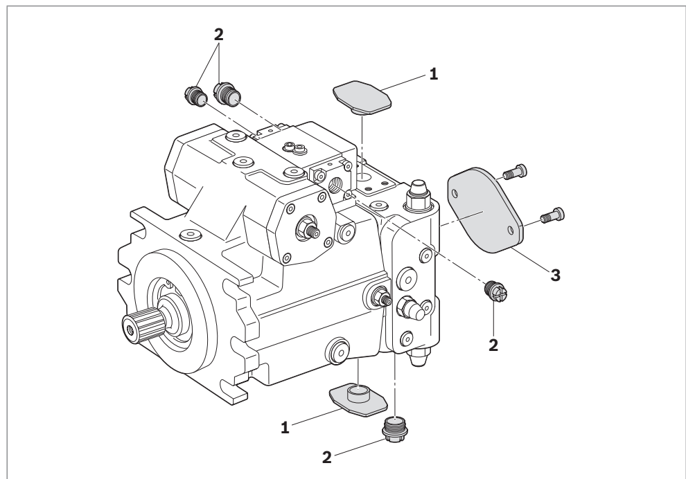
Abb. 11: Transportschutz entfernen
