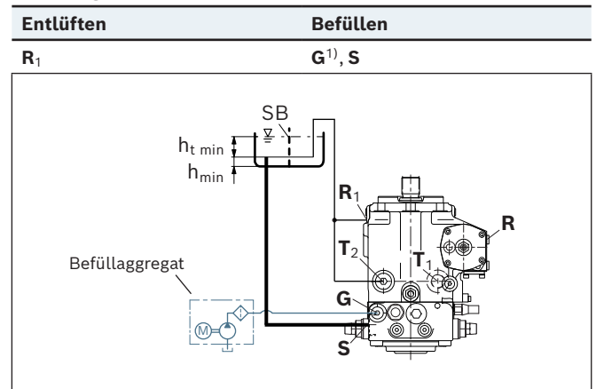
Einbaulage 4
