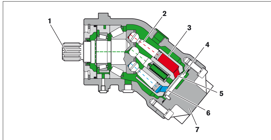
Abb. 2: Aufbau der A2FO
