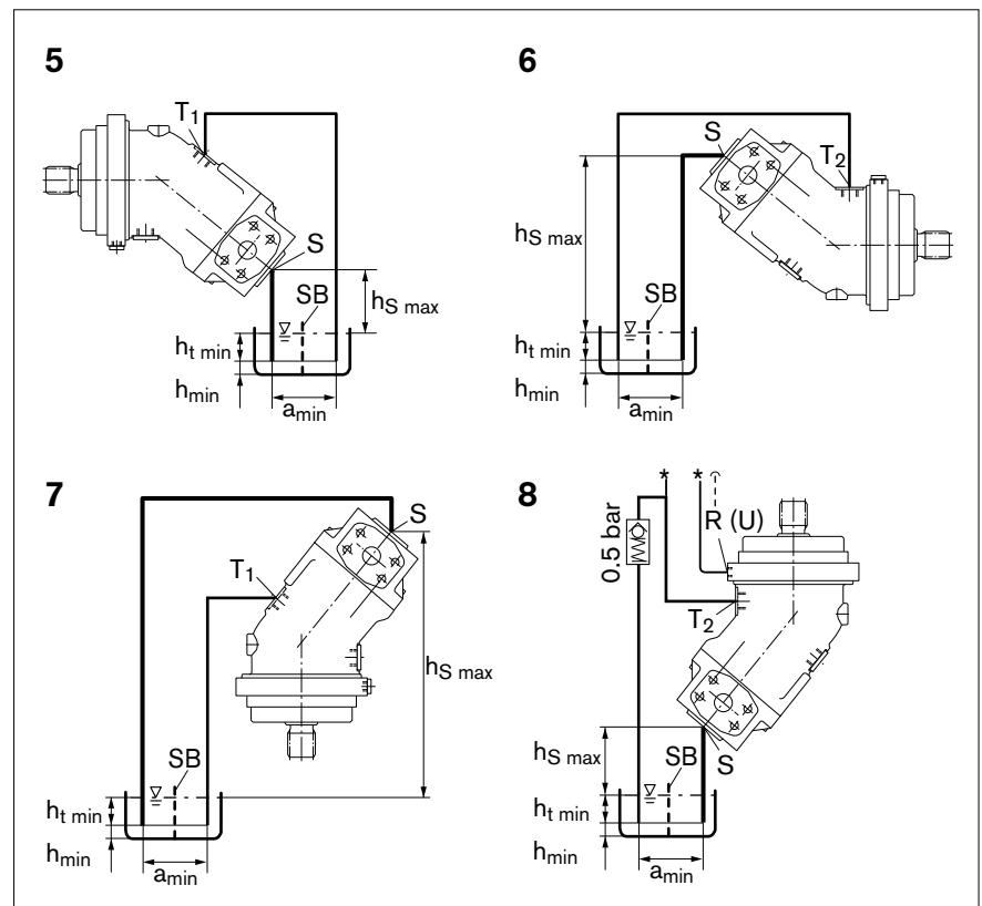
Abb. 8: Übertankeinbau A2FO mit Einbaulage 5–8
