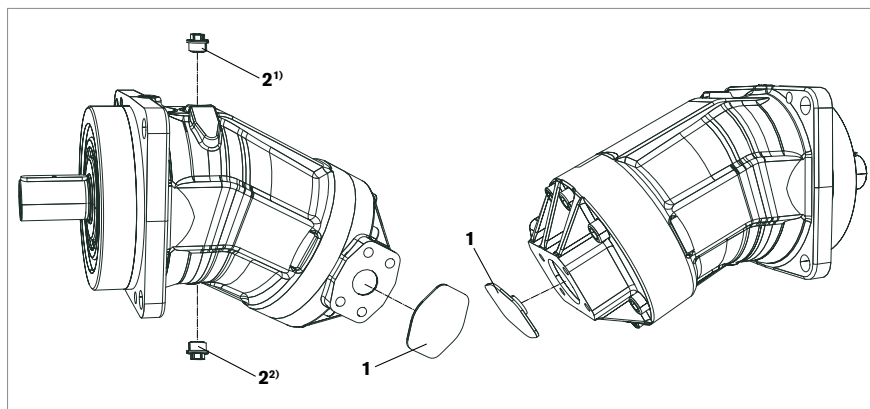
Abb. 10: Transportschutz entfernen A2FO, Nenngröße 10 bis 16
