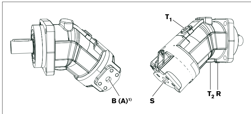
Abb. 14: Anschlussübersicht A2FO, Nenngröße 23 bis 180, Drehrichtung rechts, SAE Flanschanschlüsse seitlich/hinten (Anschlussplatte 05)
