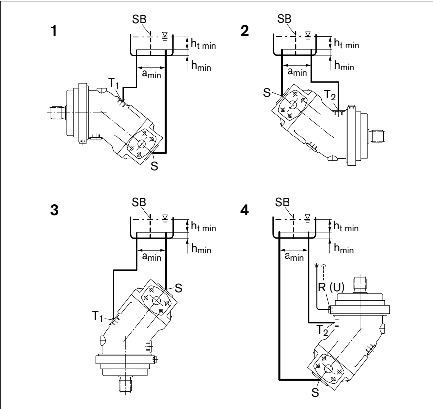
Abb. 7: Untertankeinbau A2FO mit Einbaulage 1–4
