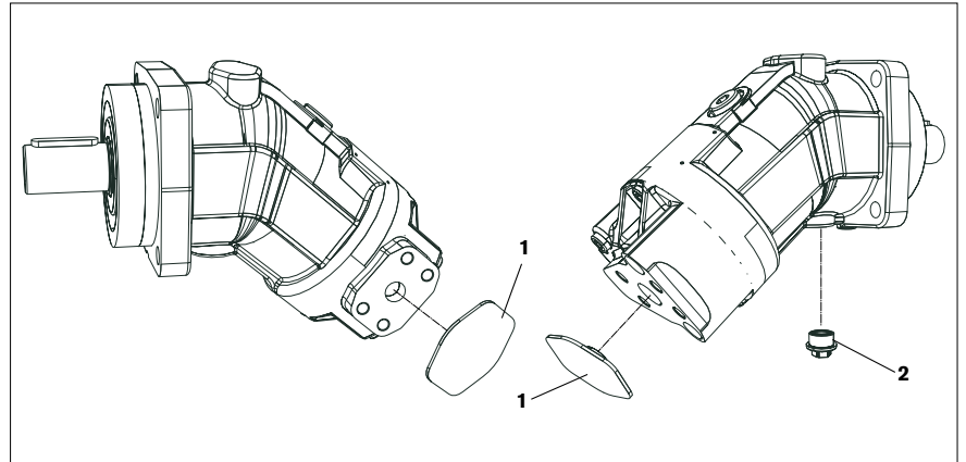
Abb. 1: Axialkolbeneinheit
