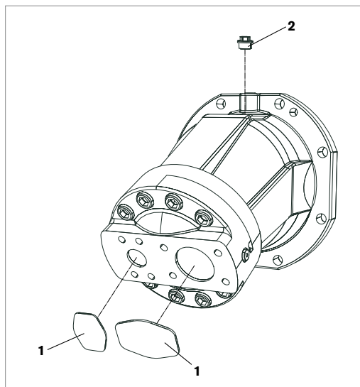
Abb. 12: Transportschutz entfernen A2FO, Nenngröße 355 bis 1000
