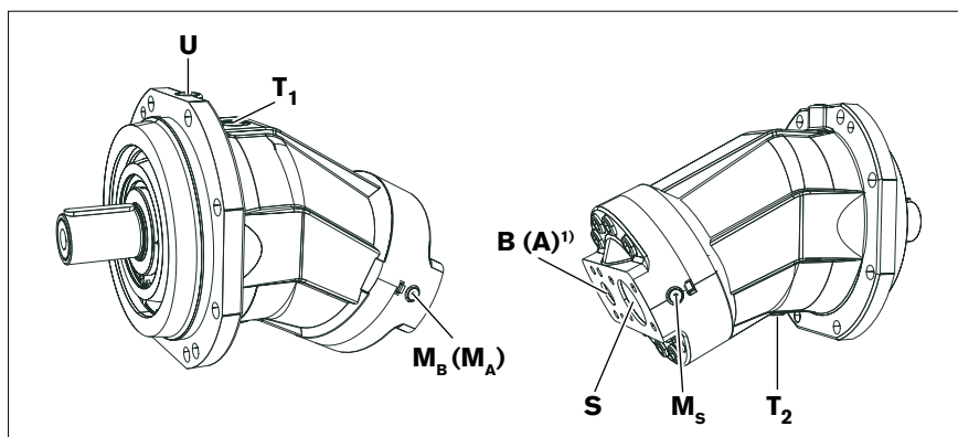
Abb. 16: Anschlussübersicht A2FO, Nenngroße 355 bis 1000, SAE Flanschanschlüsse hinten (Anschlussplatte 11)
