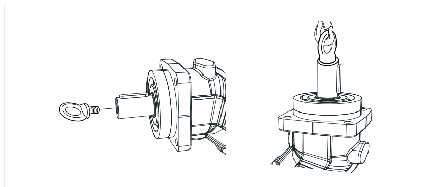
Abb. 4: Befestigung der Ringschraube
