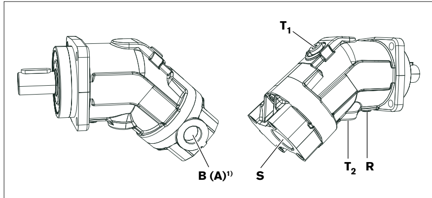
Abb. 13: Anschlussübersicht A2FO, Nenngröße 10 bis 16, Drehrichtung rechts, Gewindeanschlüsse seitlich, SAE Flanschanschluss hinten (Anschlussplatte 06)
