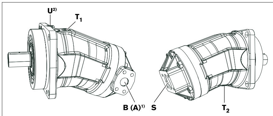
Abb. 15: Anschlussübersicht A2FO, Nenngröße 200 bis 250, Drehrichtung rechts, SAE Flanschanschluss seitlich/hinten (Anschlussplatte 05)
